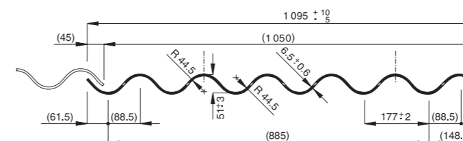
Vlnitá střešní krytina A 6,5
