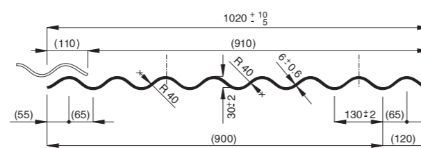
Vlnitá střešní krytina B8
