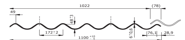
Vlnitá střešní krytina B7 CO-HO, B7 FS
