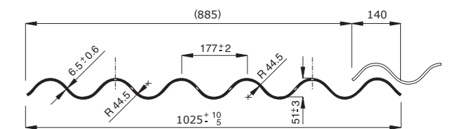
Vlnitá střešní krytina A6 CO-HO, A6 FS
