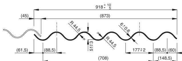
Vlnitá střešní krytina A5
